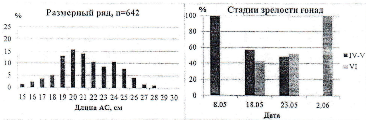
Рисунок 2 – Размерный состав и динамика стадий зрелости в скоплениях корюшки азиатской зубастой в мае 2026 г.
