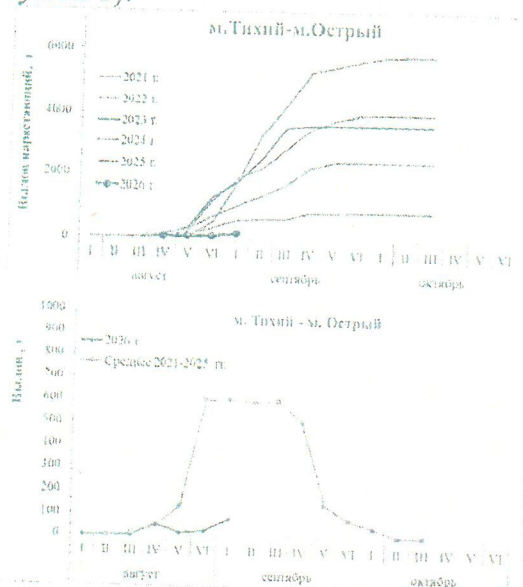
Рисунок 1 – Статистика промышленного вылова кеты на участке м. Тихий – м. Острый (по данным на 06.09.2026) (вверху кумуляты вылова, внизу приросты уловов по пятидневкам)
